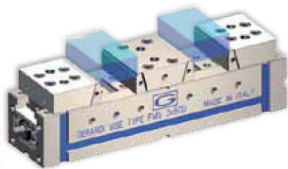
Piastre ganasce Art.806E Jaw plates Art.806E
