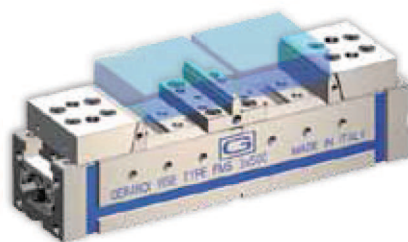
1 ganasca Art.805Q + piastre ganasce Art.806E 1 jaw Art.805Q + Jaw plates Art.806E
