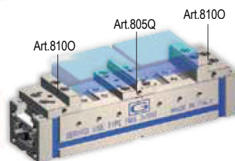
1 ganasce Art.805Q + 2 Art.8100 1 jaw Art.805Q + 2 Art.8100
