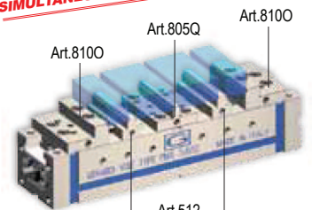
1 ganasce Art.805Q + 2 Art.8100 + 2 Art.512 1 jaw Art.805Q + 2 Art.8100 + 2 Art.512
